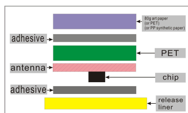
RFID label
