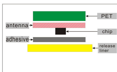
wet inlay
